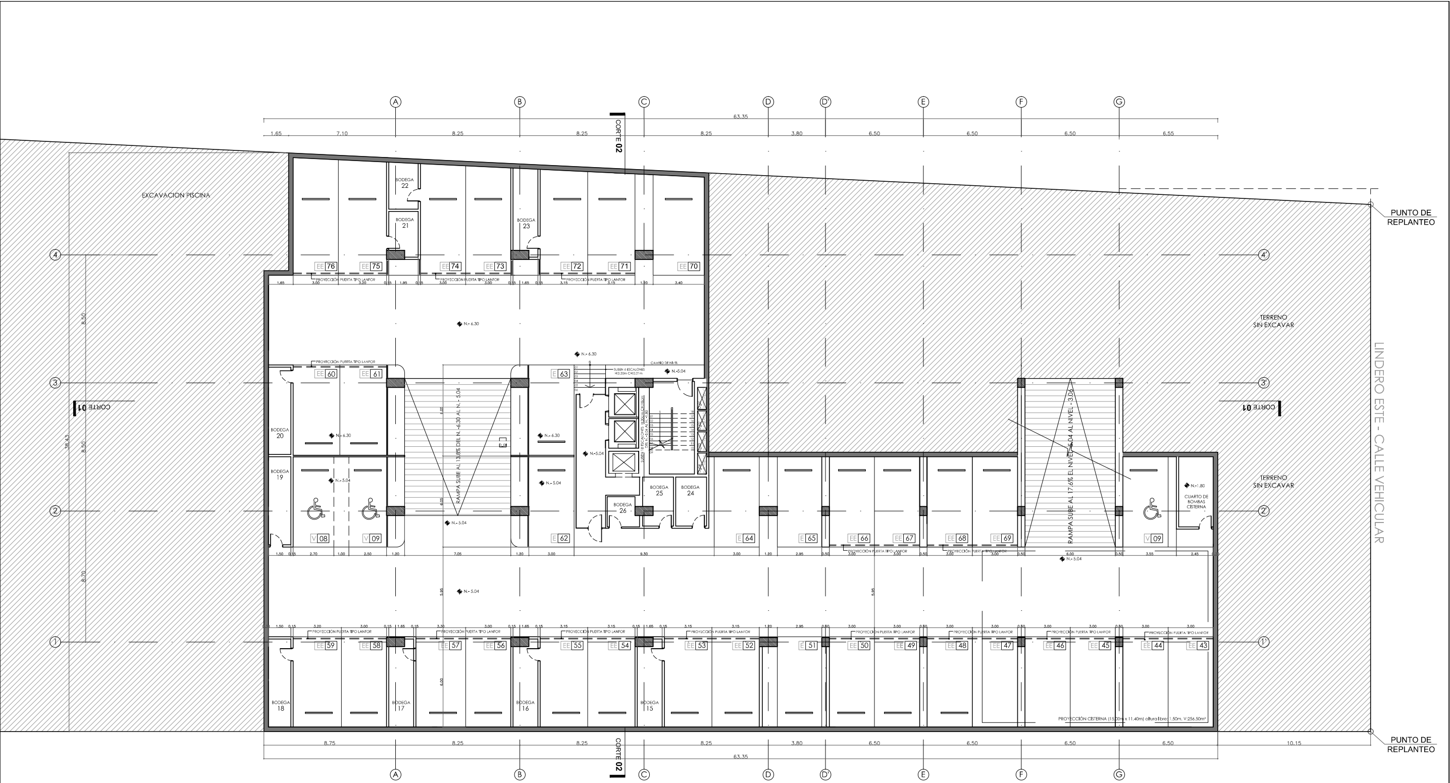
SUBSUELO 2 ESC. 1:250
